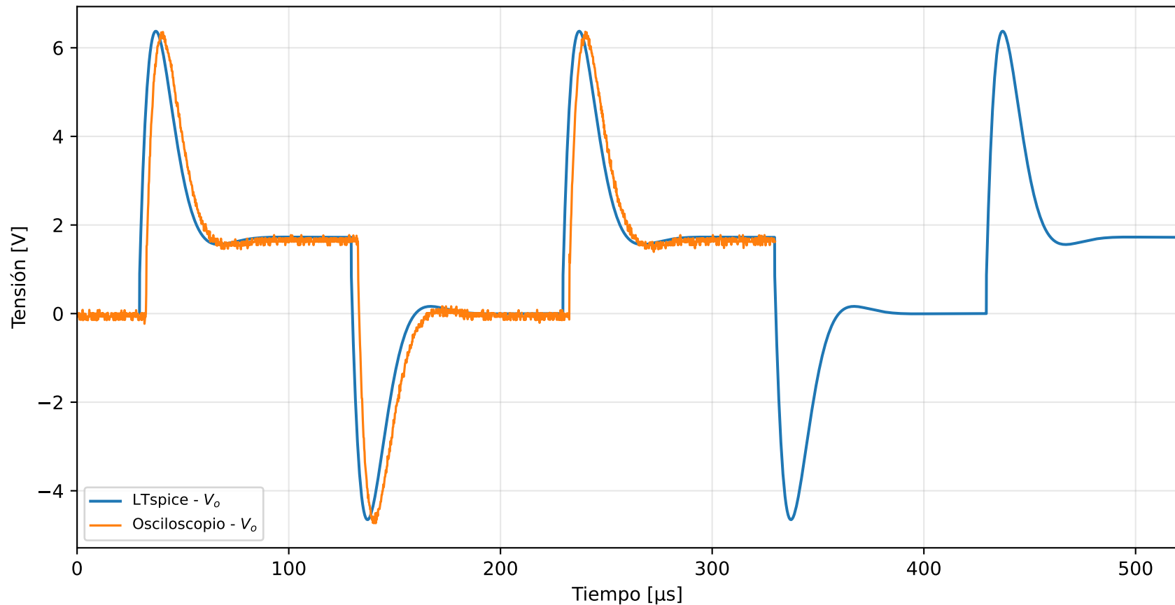
Transitorio: medición y simulación alineadas
