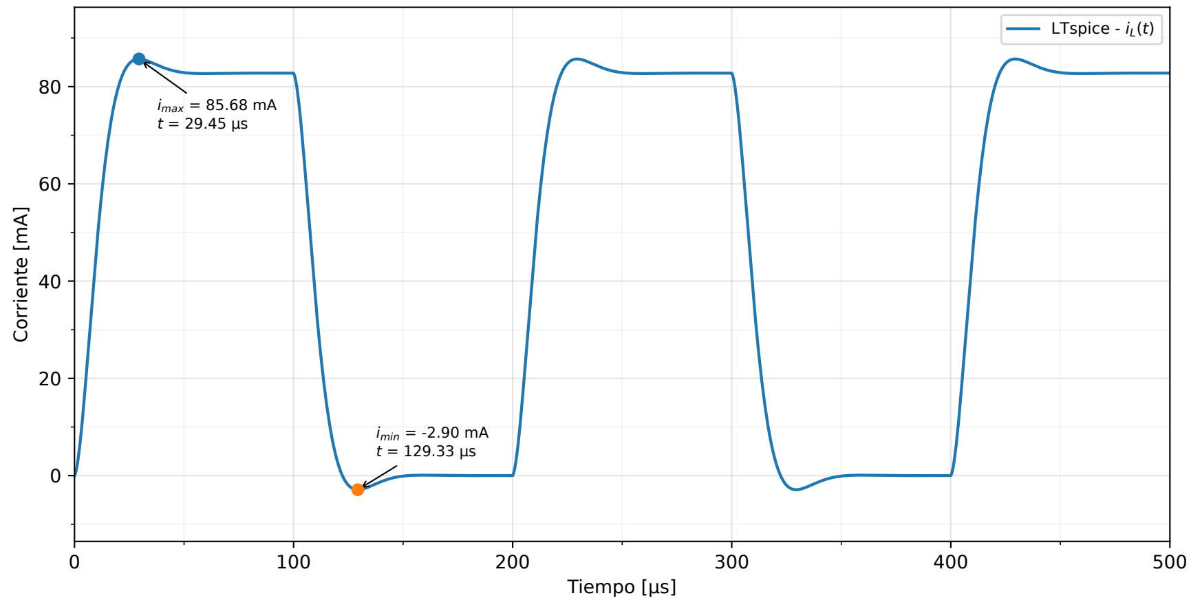
Transitorio 2.1 - corriente simulada en la bobina
