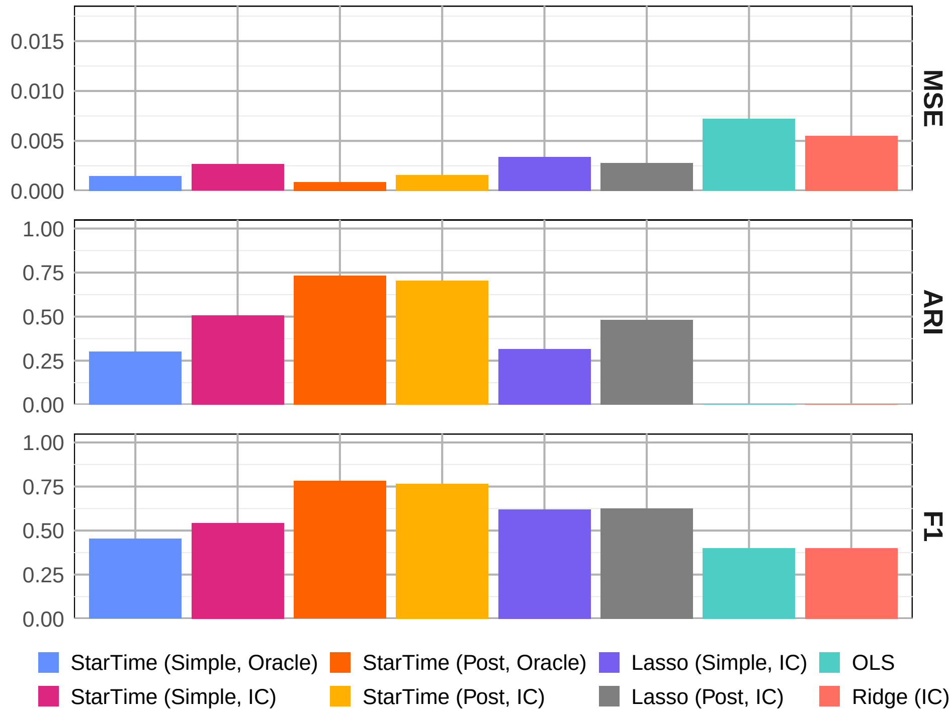
AR DGP 2, T = 200
