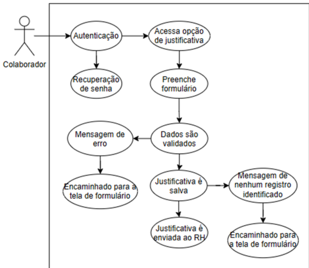
Figura 10: Caso de Uso: Enviar Justificativa por Esquecimento
