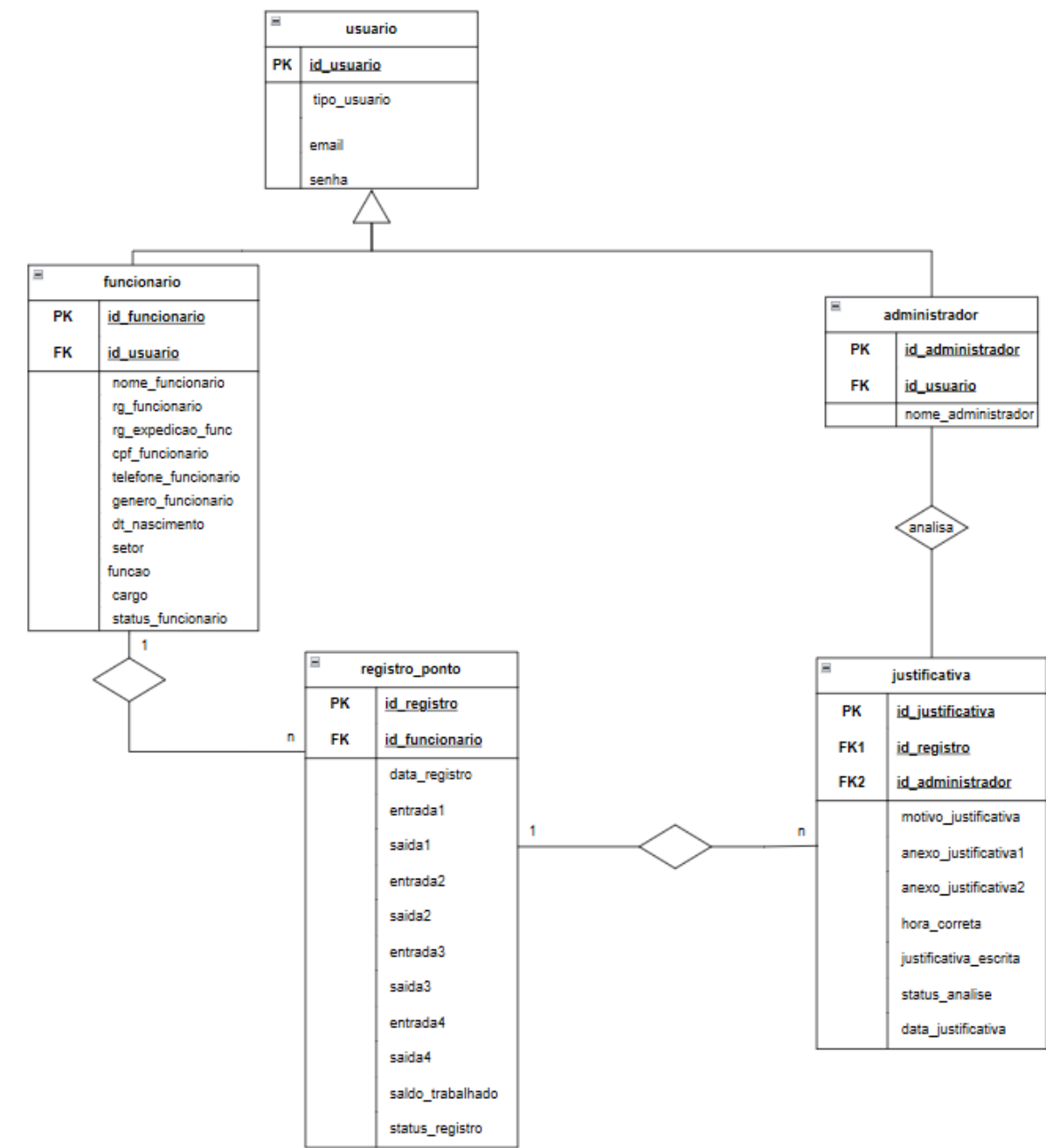
Figura 16: Modelo de Dados
