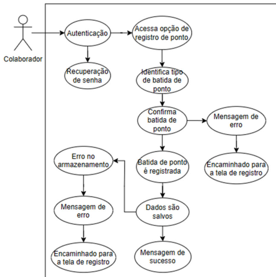
Figura 8: Caso de Uso: Registrar Batida de Ponto
