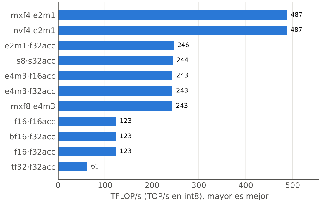
(a) Pico medido por instrucción
