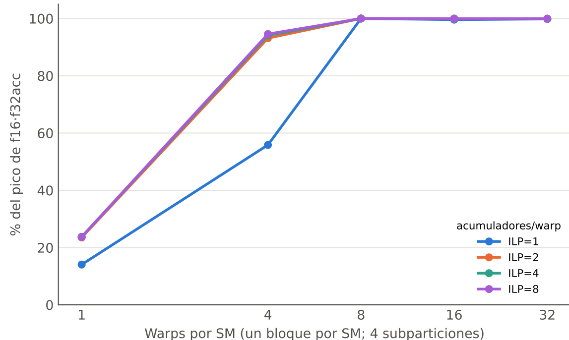
(b) Saturación (f16.f32acc): hacen falta \geq 2 warps por subpartición
