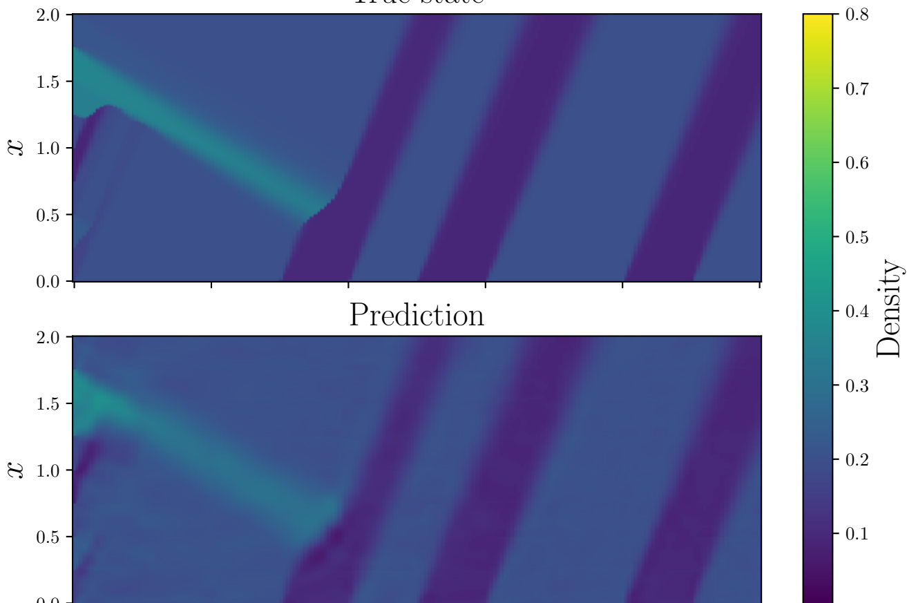
True state
