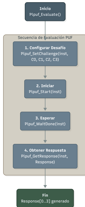
Figura 3.5: Función Plpuf_Evaluate() .
