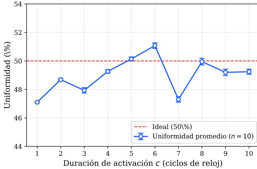
Figura 4.8: Uniformidad del PLPUF en función de la duración de activación c (media \pm 1\sigma , n = 10 ). La línea discontinua roja indica el valor ideal de 50 %.
