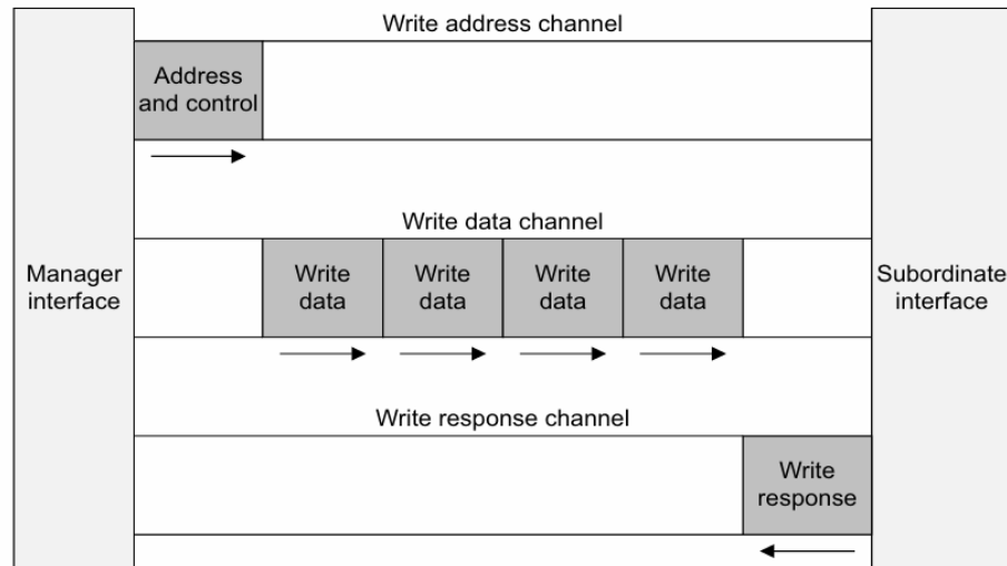
Figura 2.2: Canales de escritura del protocolo AXI: canal de dirección (AW), canal de datos (W) y canal de respuesta (B) [2].
