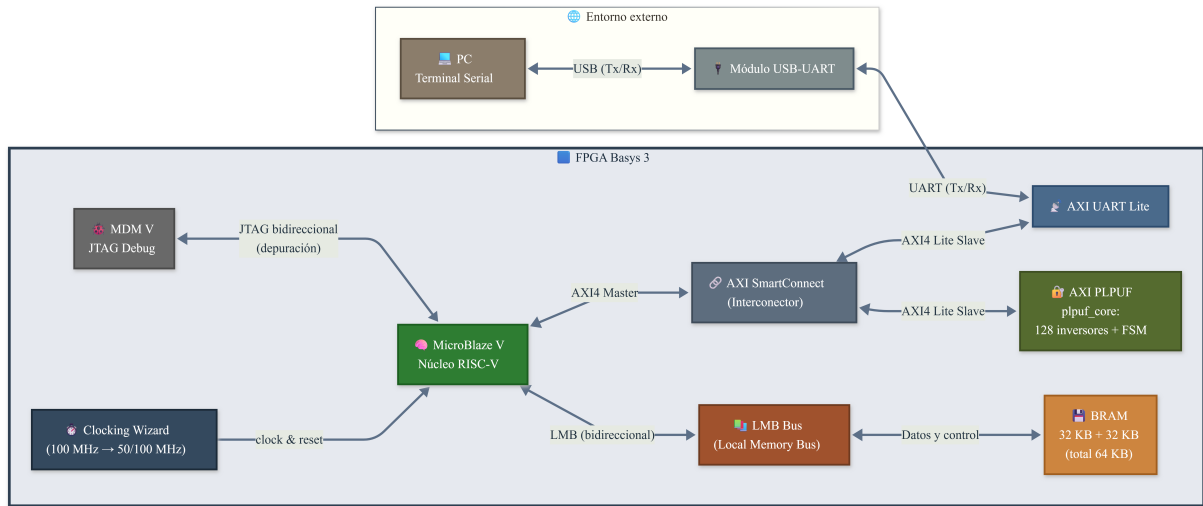
Figura 3.2: Diagrama general de la solución: sistema SoC con PLPUF integrado.
