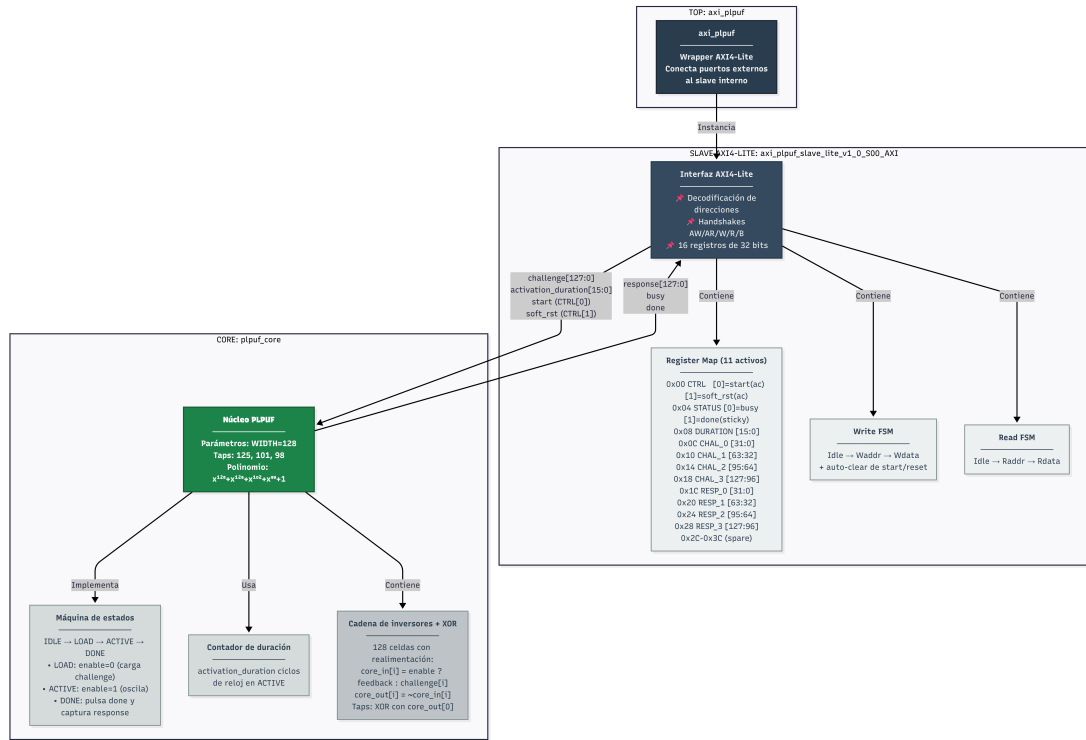
Figura 3.3: Jerarquía de módulos del IP AXI PLPUF: wrapper de nivel superior, esclavo AXI4-Lite con mapa de registros y máquinas de estado, y núcleo PLPUF con cadena de inversores, contador y FSM.
