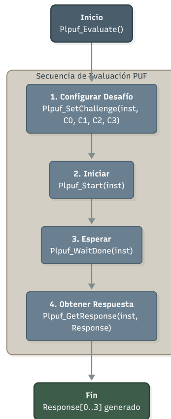
Figura 3.5: Función Plpuf_Evaluate() .
