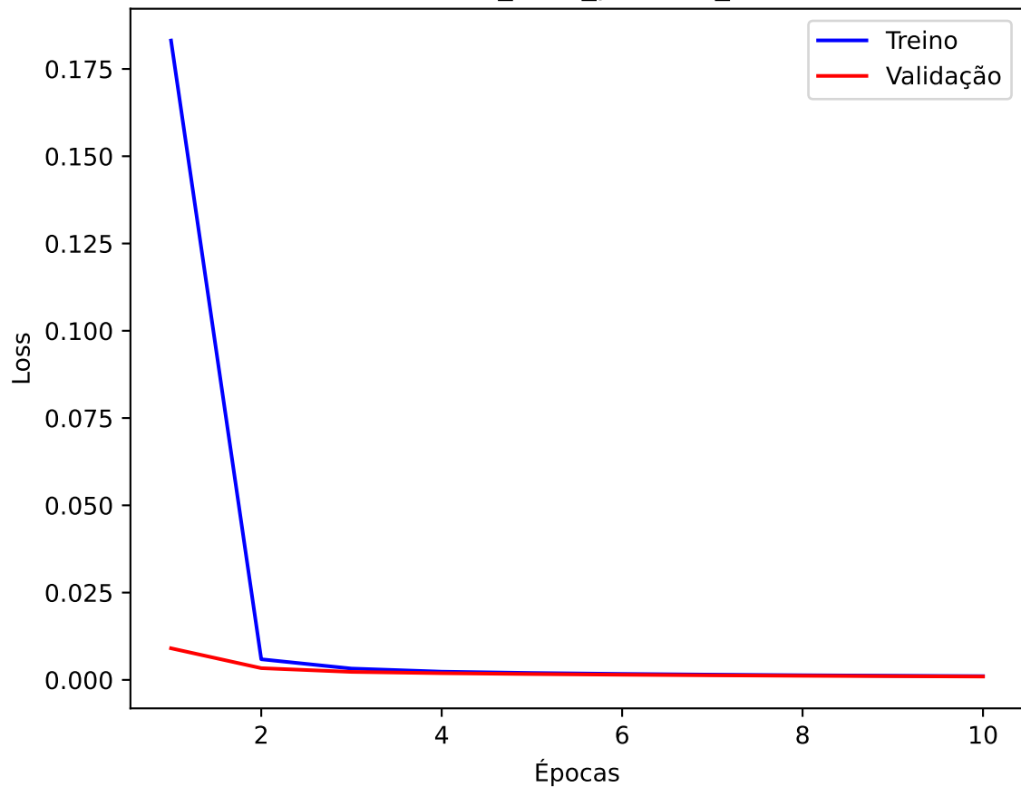
Loss - vit_base_patch16_224
