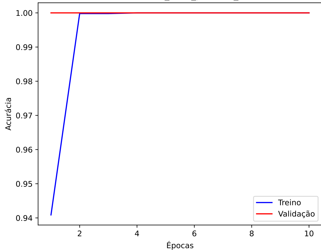
Acurácia - vit_base_patch16_224
