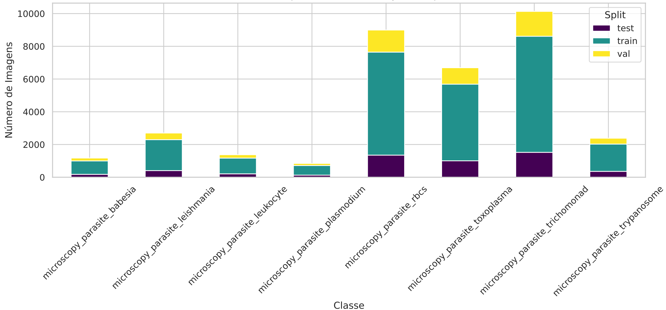
Distribuição Geral de Classes por Partição
