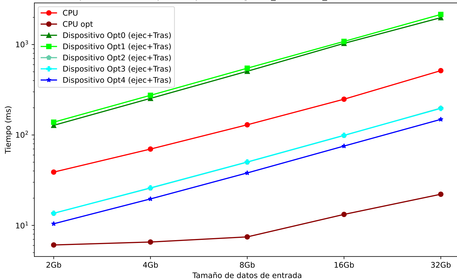
Comparación de tiempos de ejecución - global_vectorAdd_PerformanceResults.csv
