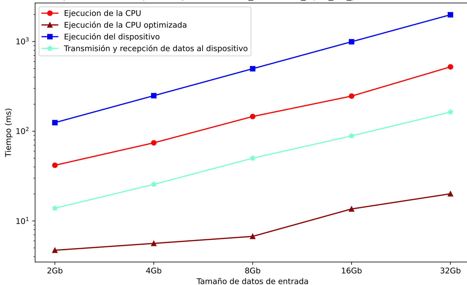
Comparación de tiempos de ejecución - test_vectorAdd_Opt1_hw_performanceResults.csv
