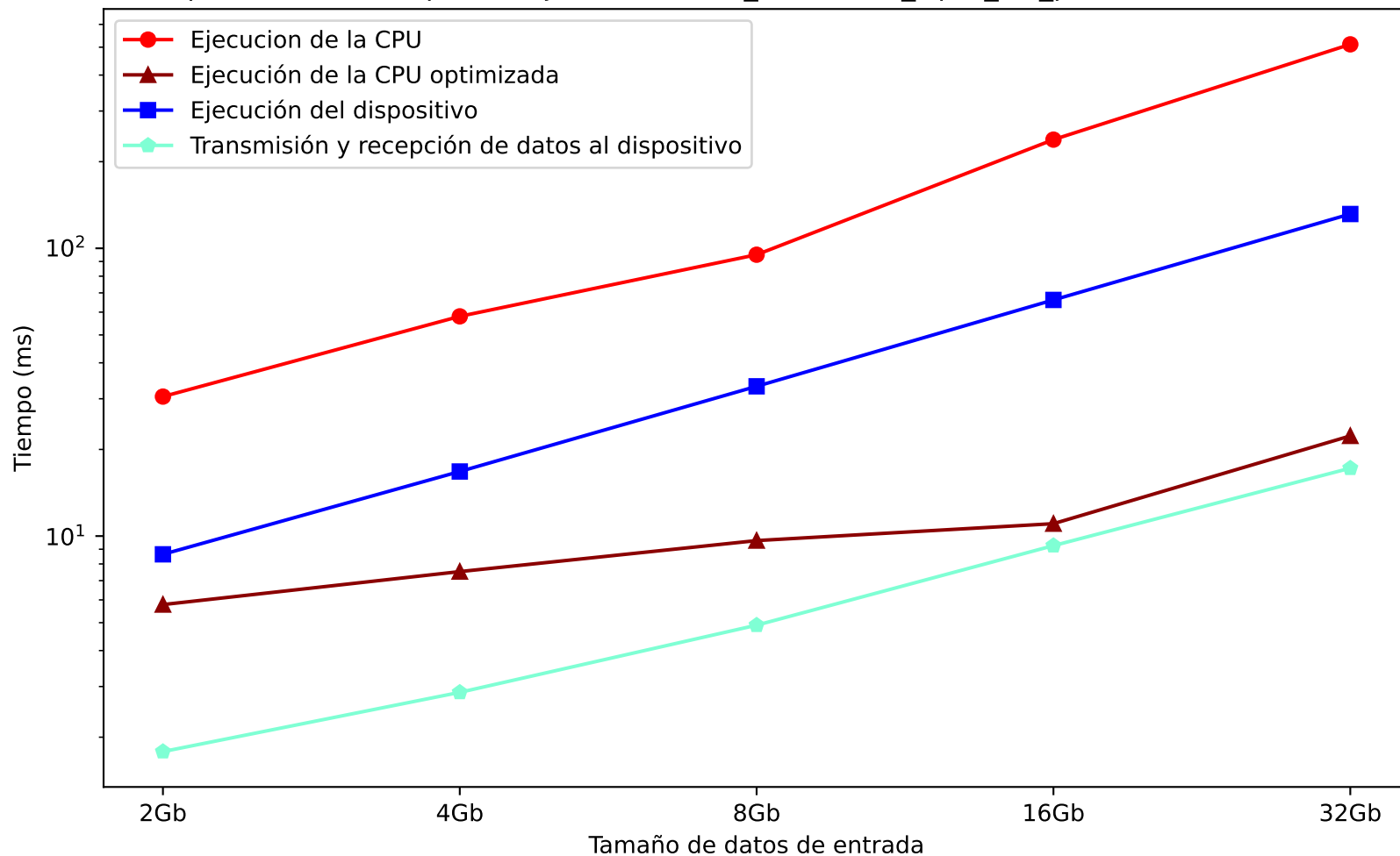
Comparación de tiempos de ejecución - test_vectorAdd_Opt4_hw_performanceResults.csv
