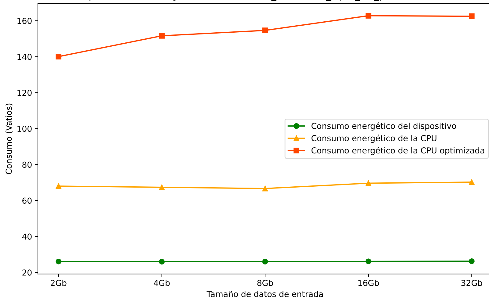
Comparación de energía consumida - test_vectorAdd_Opt0_hw_powerResults.csv
