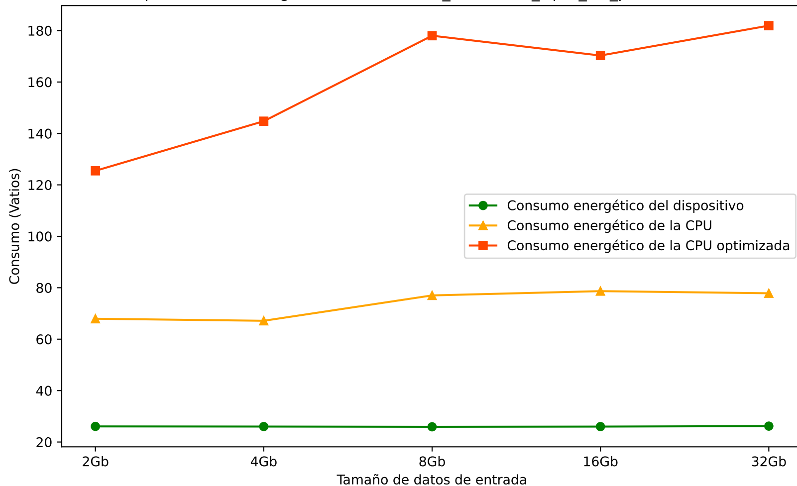
Comparación de energía consumida - test_vectorAdd_Opt1_hw_powerResults.csv
