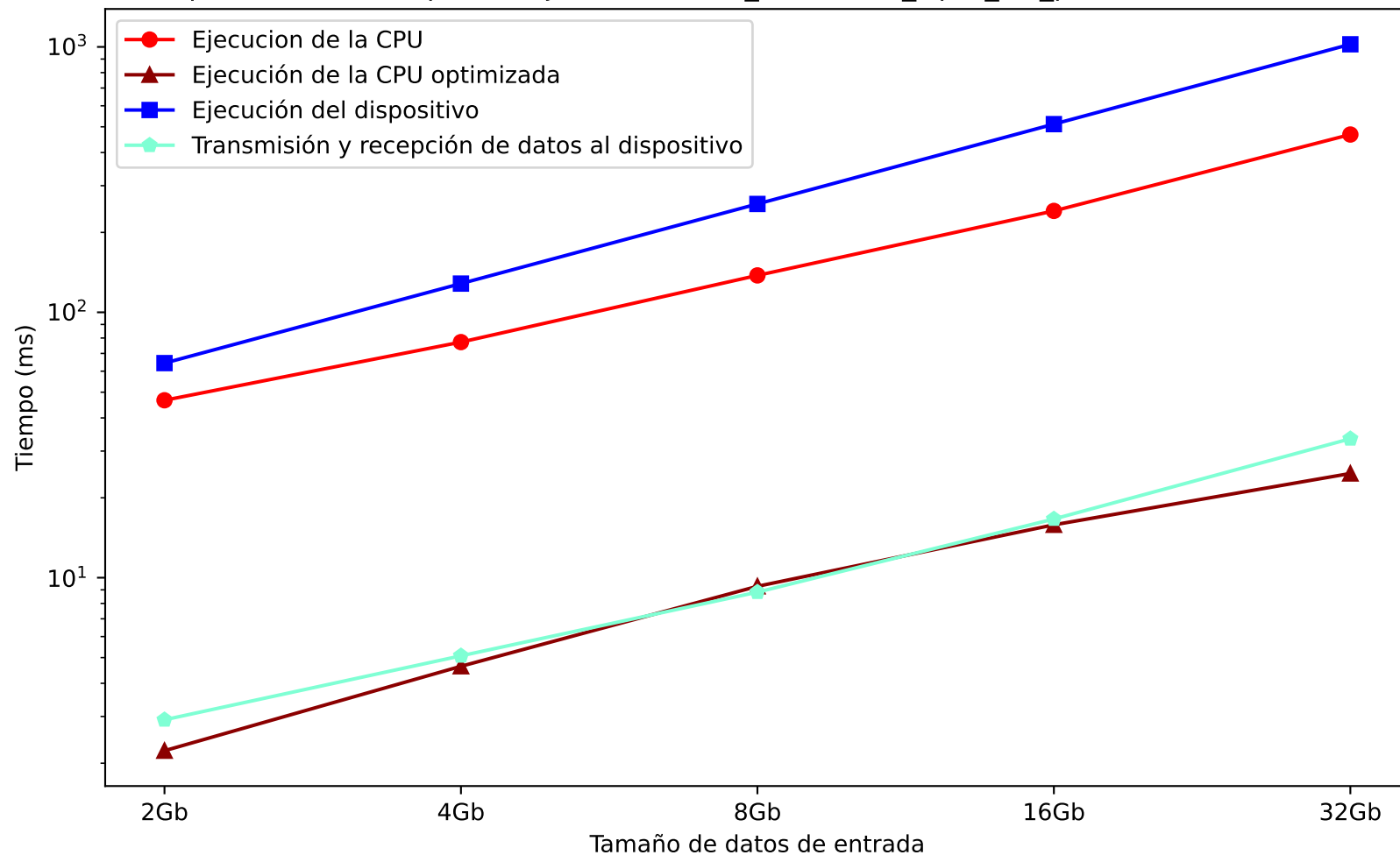
Comparación de tiempos de ejecución - test_vectorAdd_Opt2_hw_performanceResults.csv
