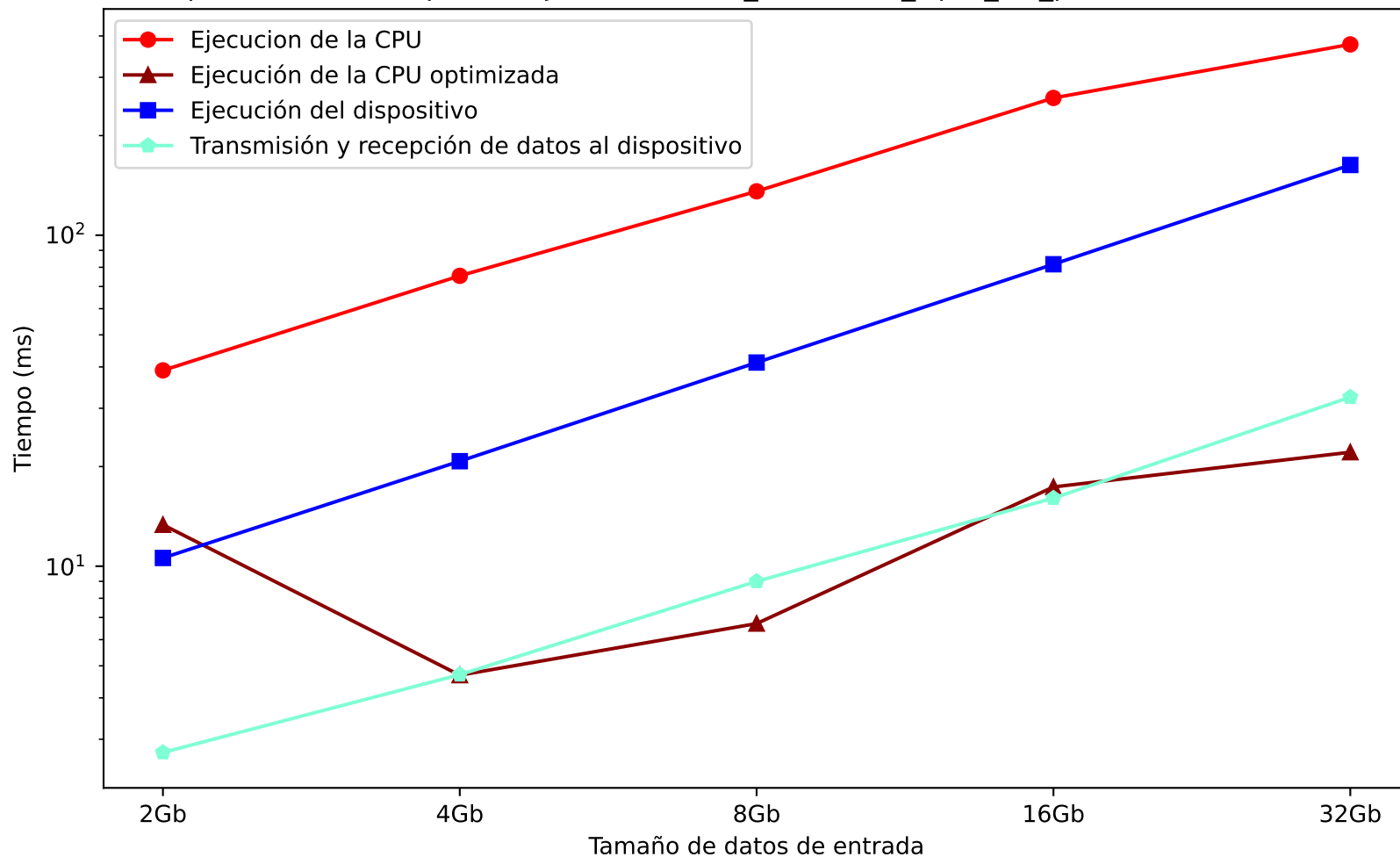
Comparación de tiempos de ejecución - test_vectorAdd_Opt3_hw_performanceResults.csv
