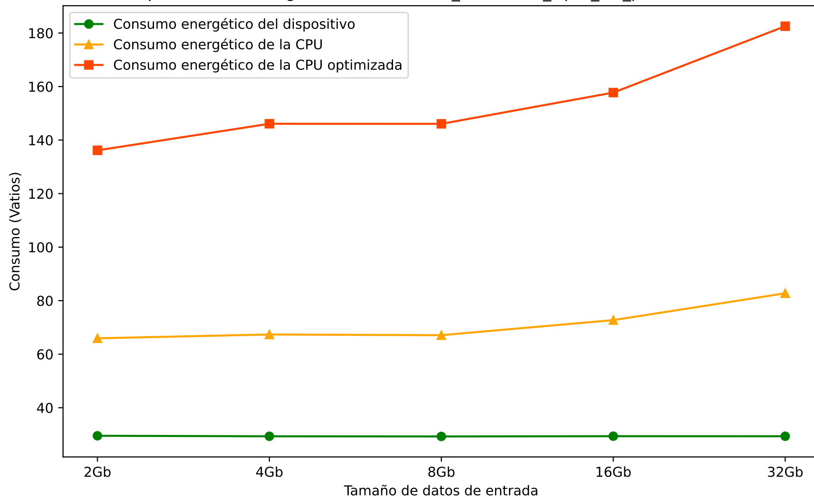
Comparación de energía consumida - test_vectorAdd_Opt3_hw_powerResults.csv
