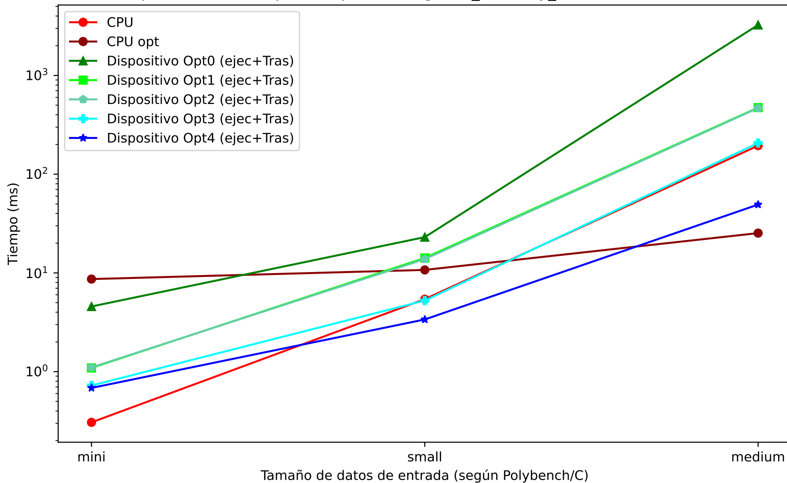
Comparación de tiempos de ejecución - global_cholesky_PerformanceResults.csv
