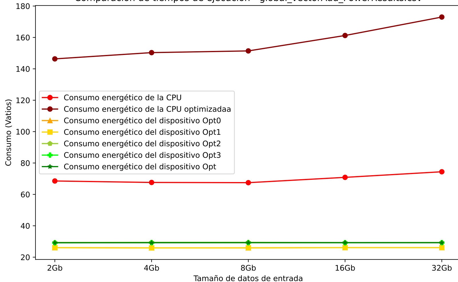
Comparación de tiempos de ejecución - global_vectorAdd_PowerResults.csv
