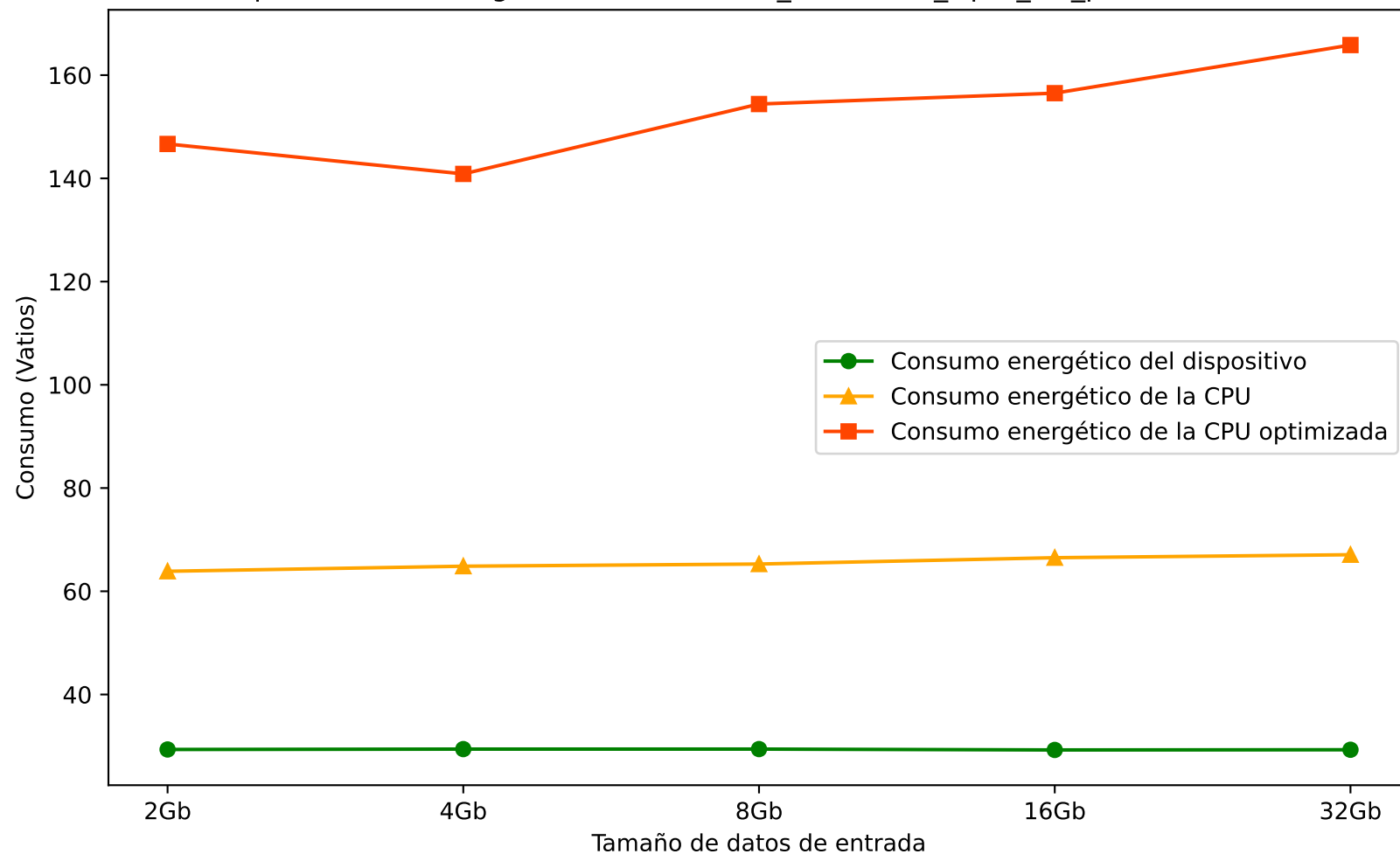
Comparación de energía consumida - test_vectorAdd_Opt2_hw_powerResults.csv
