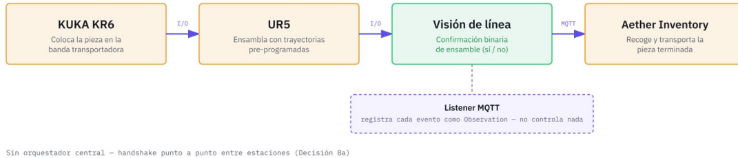
Figura 8. Línea de manufactura – enlace punto a punto entre estaciones.
