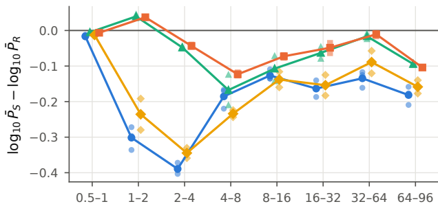
OASIS-1 T1
