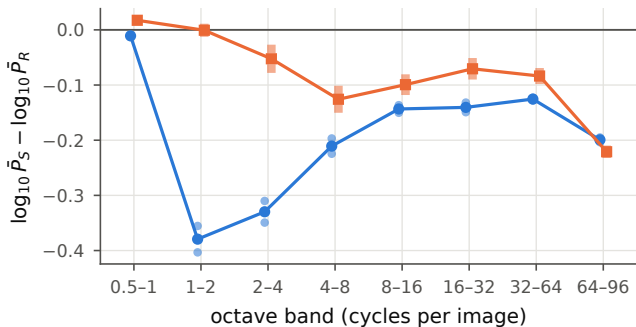
OASIS-1 T1
