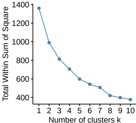
Numero optimo de clusters
