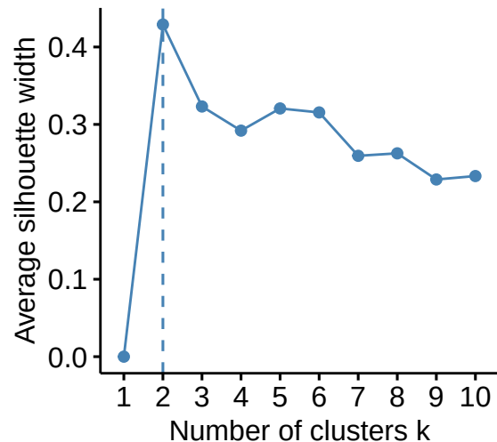
Numero optimo de clusters
