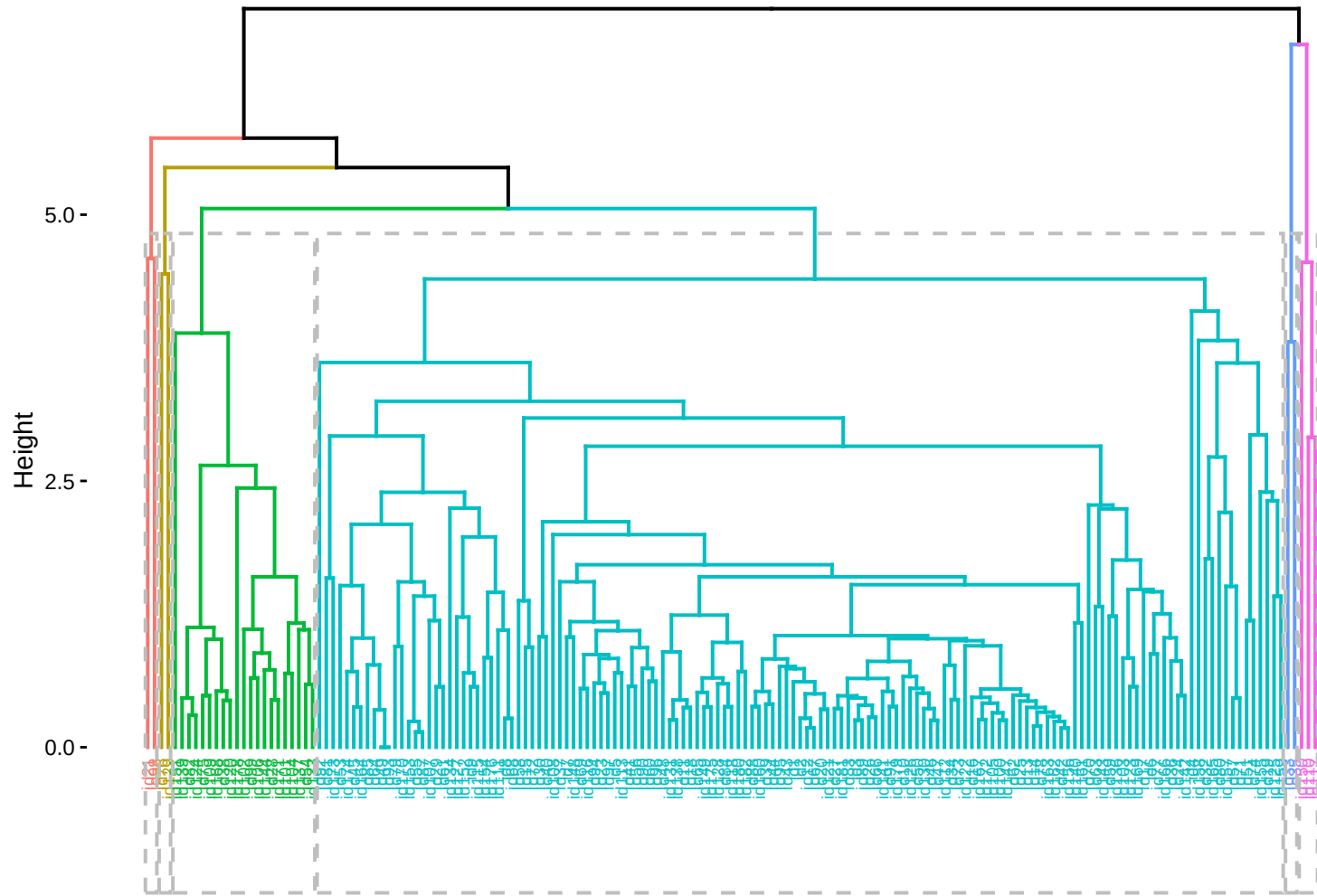
Dendrograma — Método: average
