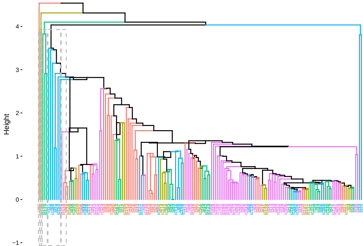
Dendrograma — Método: centroid
