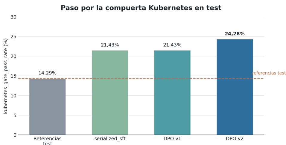
Figura 8.2: Comparación de la kubernetes_gate_pass_rate en test entre las referencias del split y las variantes más fuertes de la rama serializada. La compuerta corresponde al nivel final de la métrica KDV automática
