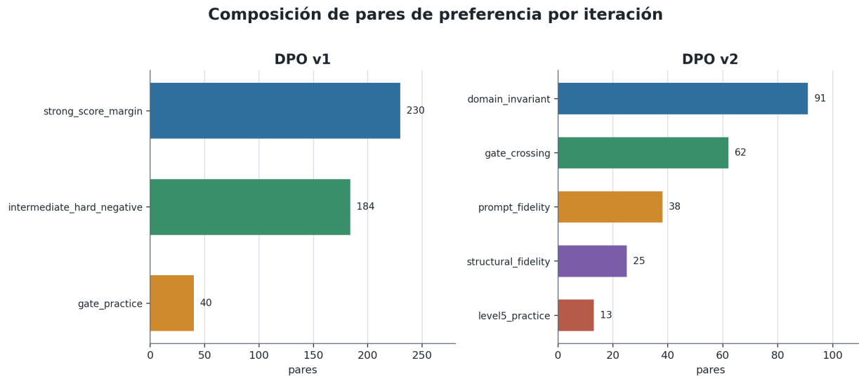
Figura 7.6: Composición de tipos de pares en DPO v1 y DPO v2. La segunda iteración reduce el número total de pares, pero desplaza el foco hacia contrastes más específicos de dominio y estructura.
