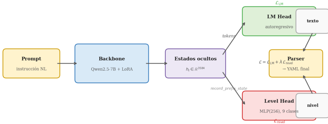
Arquitectura two-head: cabezal de lenguaje y cabezal de nivel explícito
