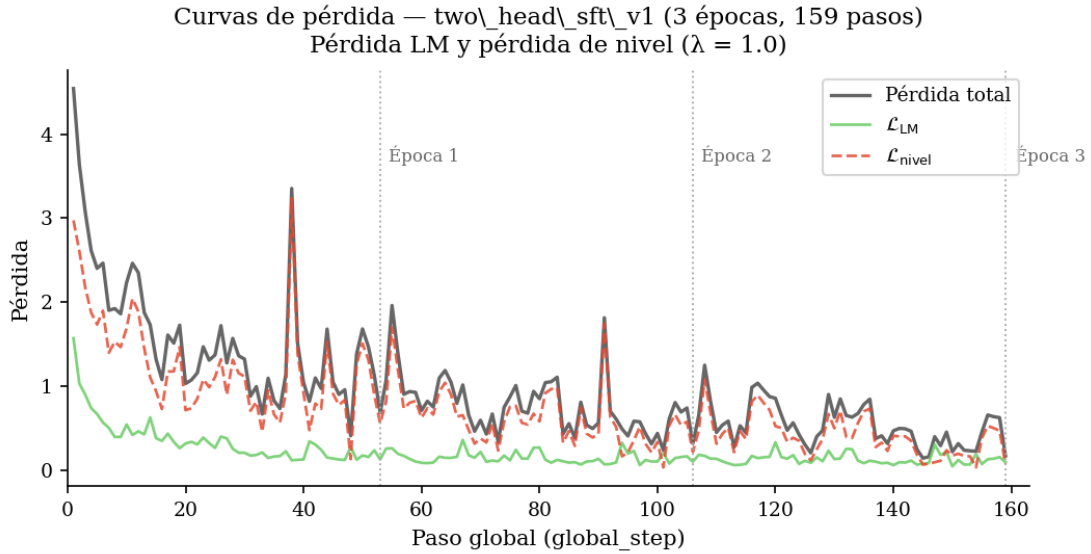
Figura 6.3: Curvas de pérdida durante el entrenamiento del THM v1: pérdida total, componente LM y componente de nivel ( \lambda = 1.0 , 3 épocas, 159 pasos globales).
