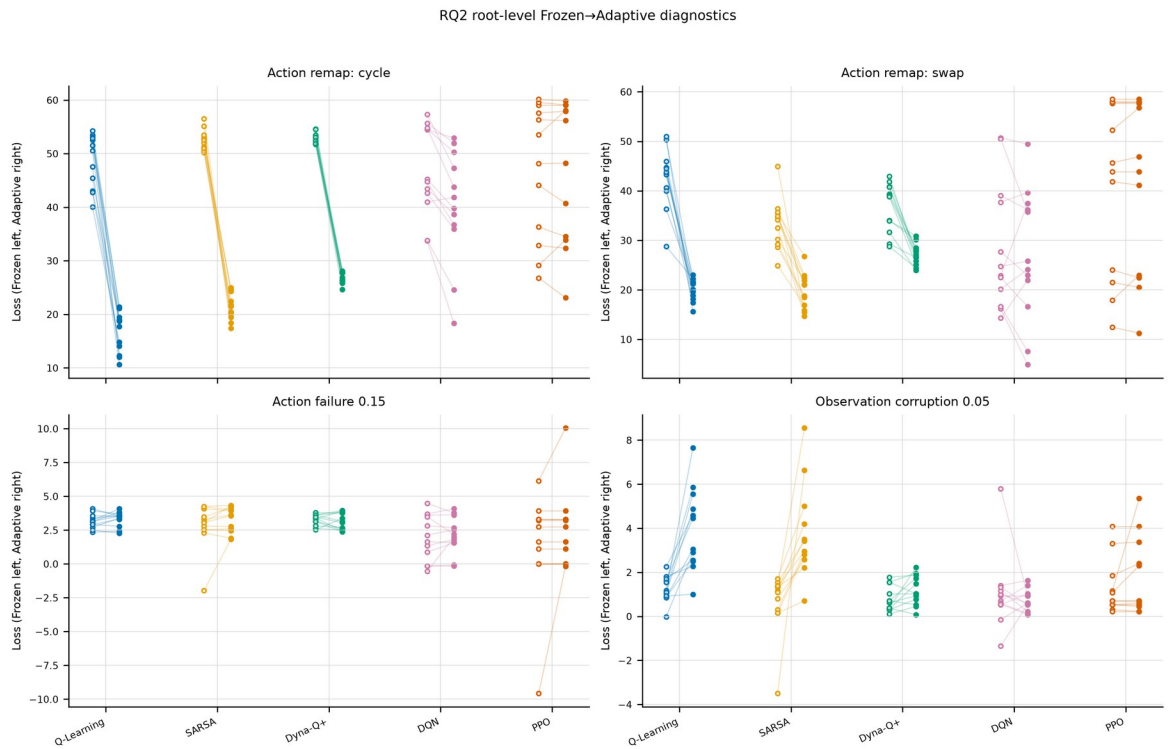
Σχήμα 18 — Όλες οι προκαθορισμένες paired συγκρίσεις A-B του RQ2 ανά συνθήκη και estimand.
