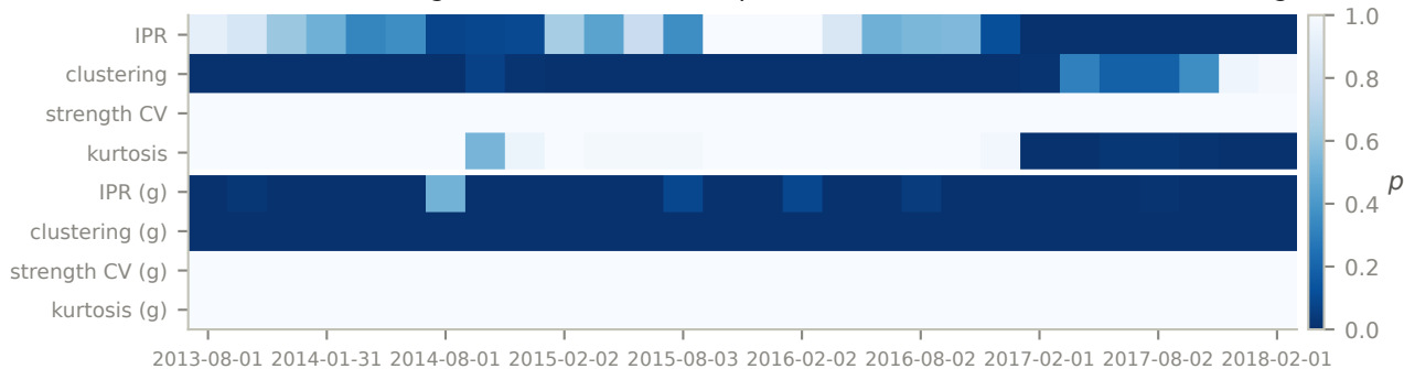
(d) S&P 500 rolling windows: conditional p -values (raw / after Gaussianization ``g'')
