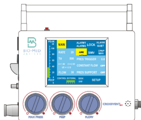
FIG. 1- VISTA FRONTAL
