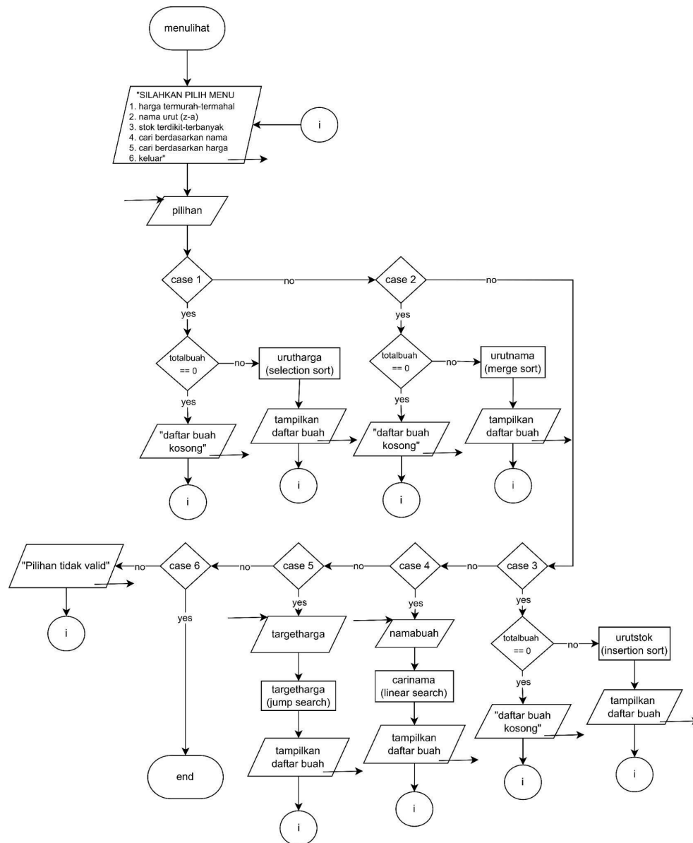
Gambar 2.17.1 flowchart menulihat
