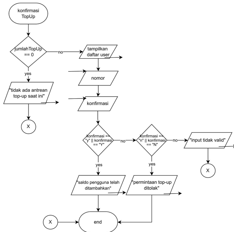
Gambar 2.11.1 flowchart konfirmasiTopUp
