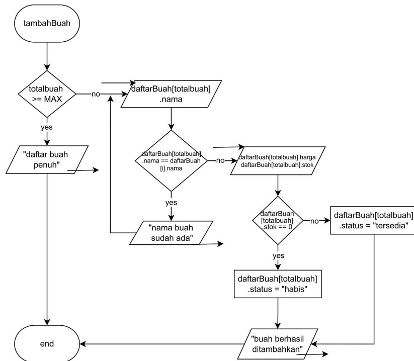
Gambar 2.7.1 flowchart tambahBuah
