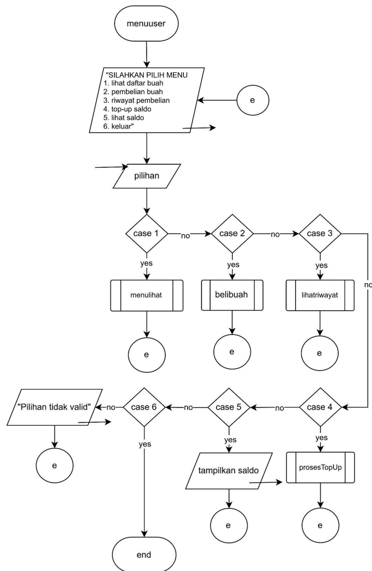
Gambar 2.13.1 flowchart menuuser
