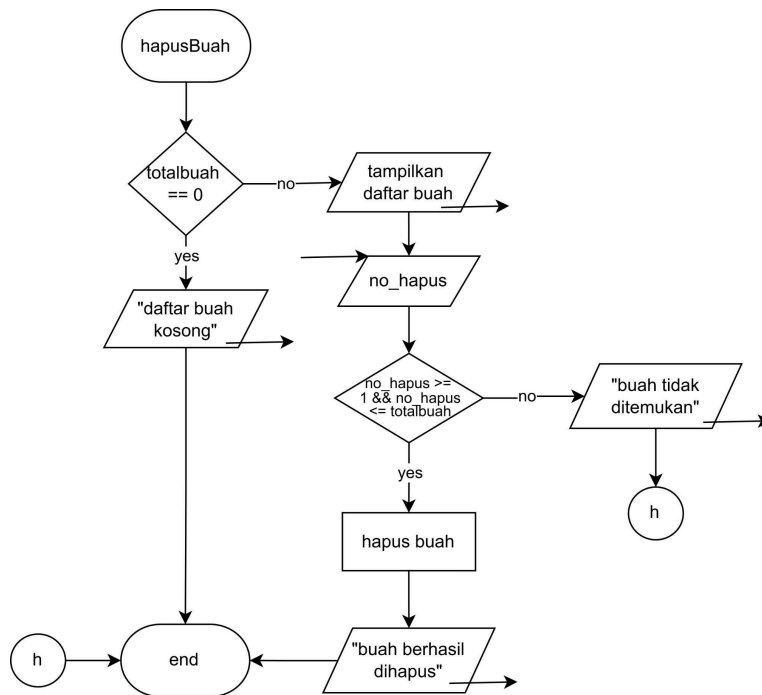
Gambar 2.9.1 flowchart hapusBuah
