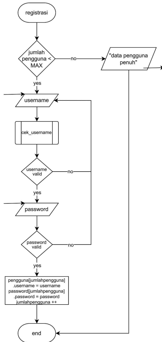
Gambar 2.5.1 flowchart registrasi
