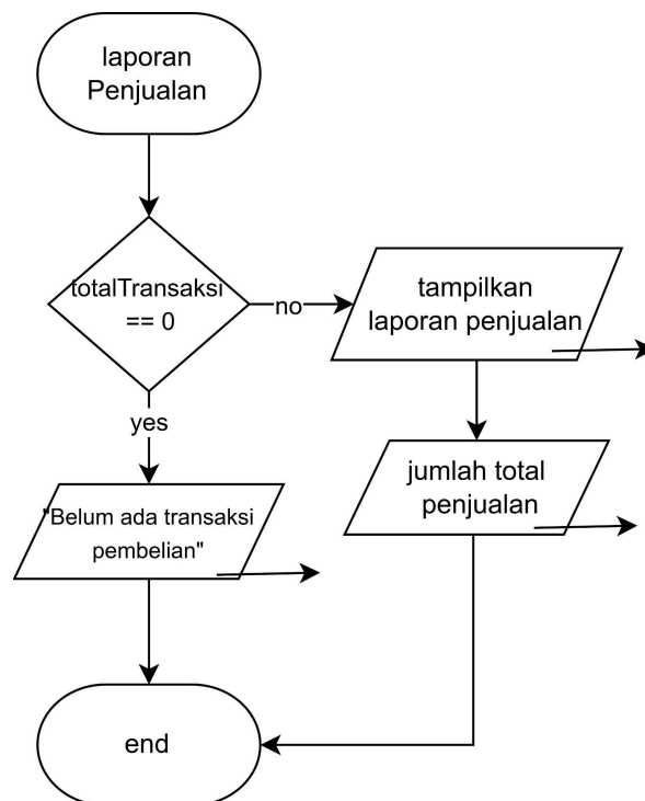
Gambar 2.10.1 flowchart laporanPenjualan
