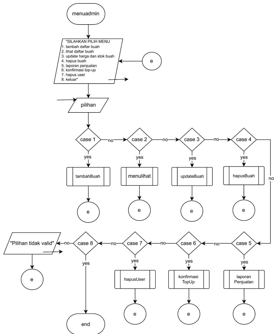
Gambar 2.6.1 flowchart menuadmin
