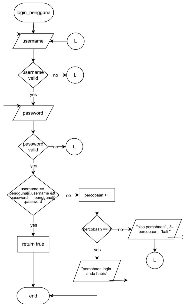
Gambar 2.3.1 flowchart login_pengguna
