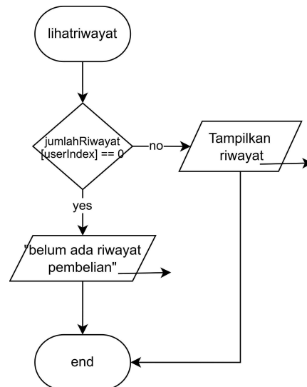
Gambar 2.15.1 flowchart lihatriwayat
