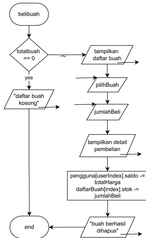
Gambar 2.14.1 flowchart belibuah
