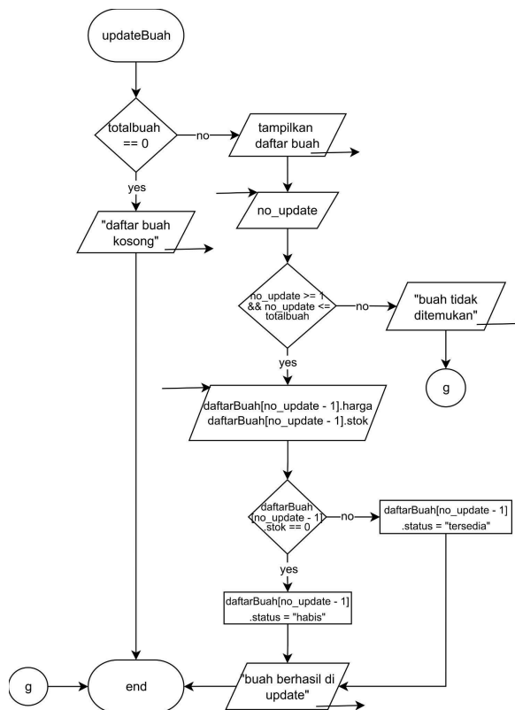
Gambar 2.8.1 flowchart updateBuah
