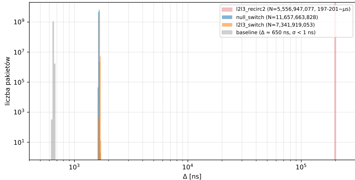
\Delta_{\text{DUT}} vs \Delta_{\text{baseline}} -- 3 programy DUT (15 min)
