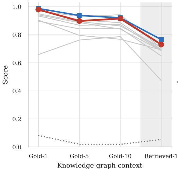
Answer-set F1
