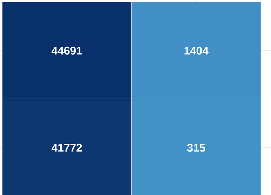
Matriz de confusión – Modelo final (Regresión Logística)
