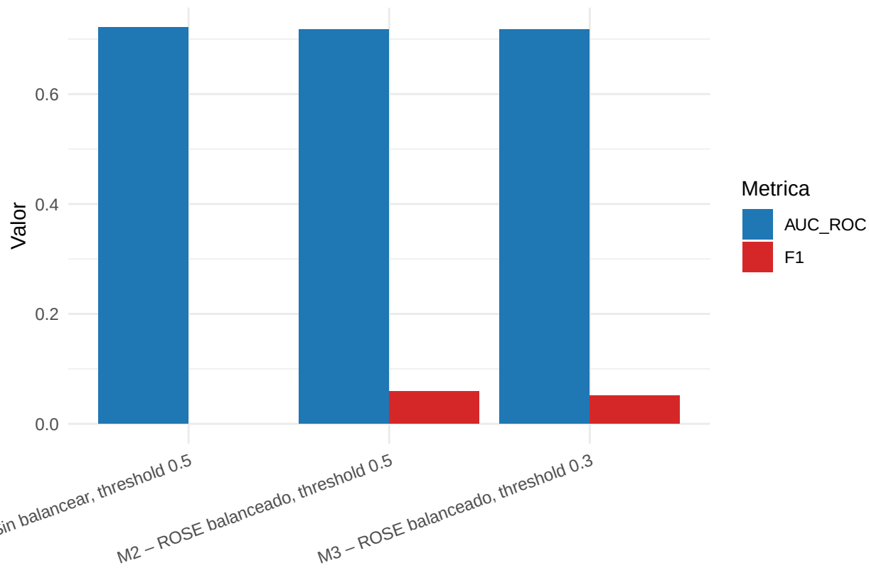
Comparación de modelos – F1 y AUC-ROC
