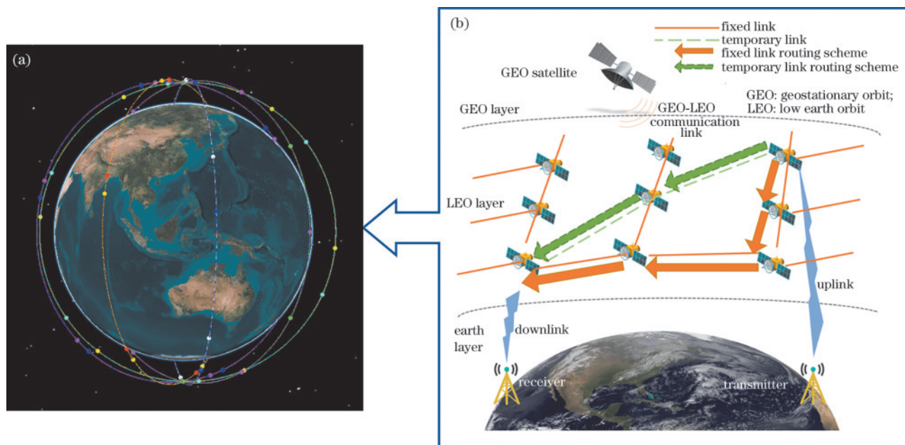
图3 星间激光通信路由链路图。(a)Systems Tool Kit搭建的星座;(b)固定链路与时空链路对比图
