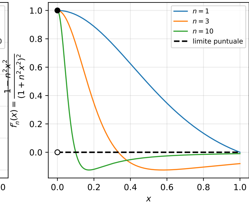
Le derivate convergono solo puntualmente
