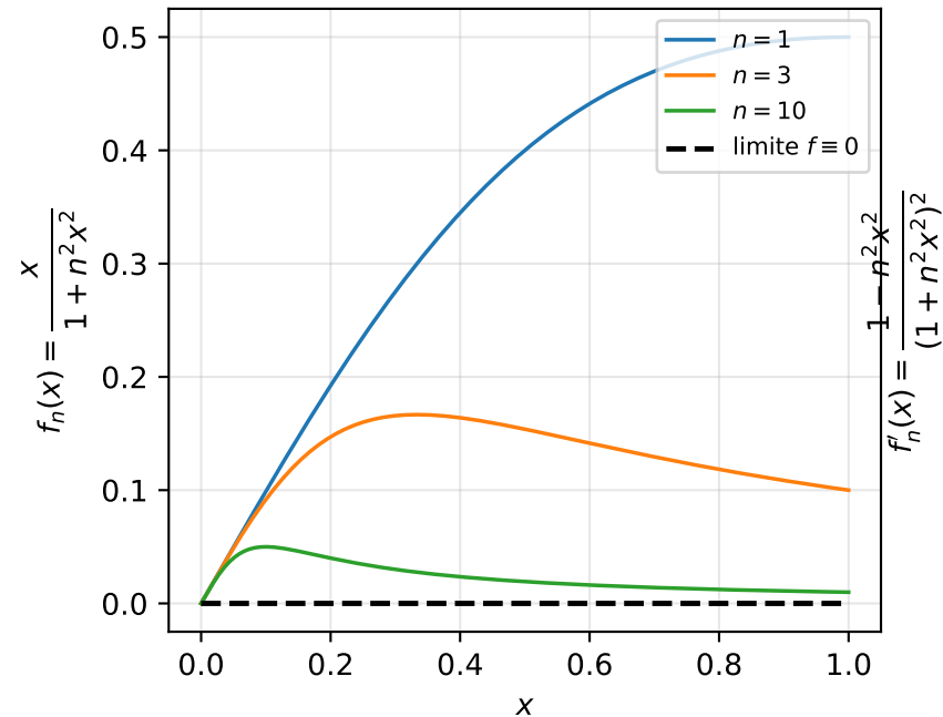
Convergenza uniforme a f \equiv 0
