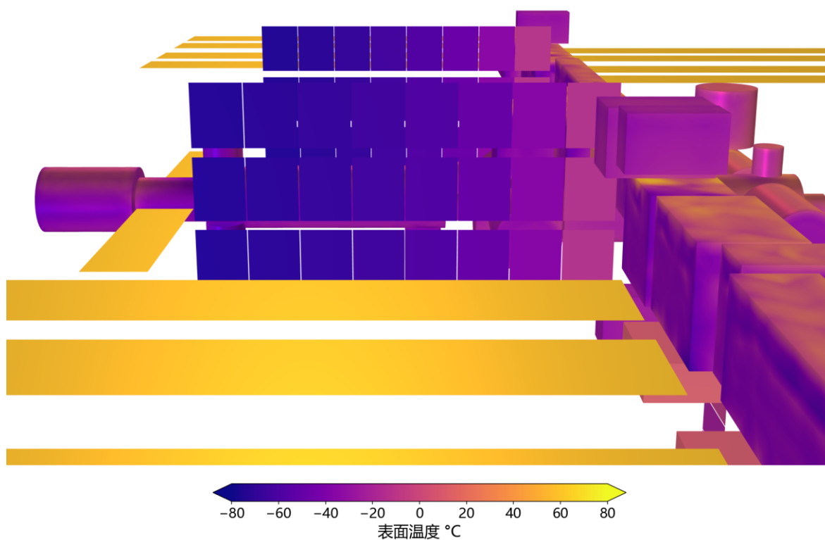
图 11 设计冷工况第三圈正午右舷 EATCS 散热器翼的表面温度，自右舷上方观察，最上一排为后方左舷翼的面板，前景横条为右舷太阳翼
