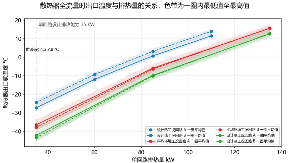
图 23 散热器全流量时出口氨温度与单回路排热量的关系
