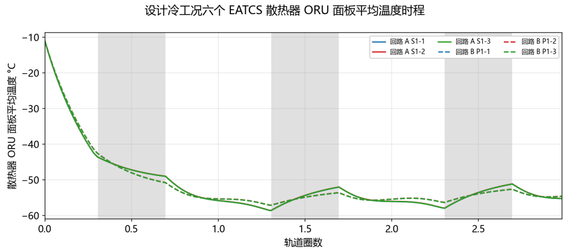
图 8 设计冷工况下六个 EATCS 散热器 ORU 面板平均温度时程，同一翼三个 ORU 的曲线基本重合
