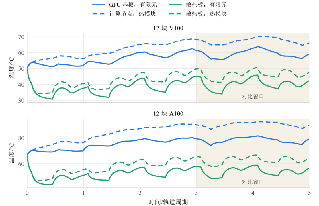
图 3 FE-004 GPU 基板、计算节点与散热板温度时程
