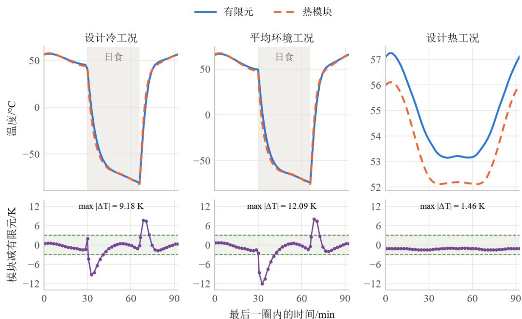
图 1 FE-001 太阳能板最后一圈温度对比
