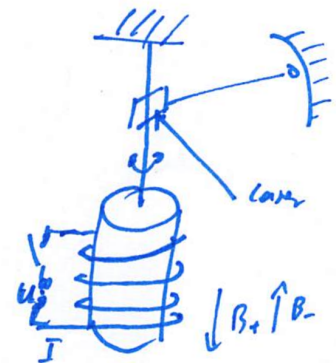
Abbildung 7.1: Einstein-de Haas-Experiment
