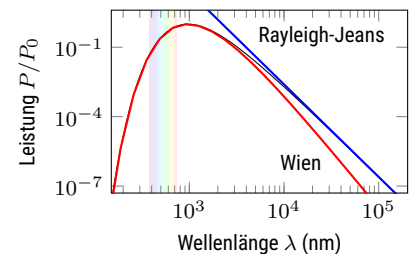
Abbildung 1.1: Schwarzkörperspektren. Oben: lineare Darstellung für T = 3000 \text{ K} , 4000 \text{ K} und 5000 \text{ K} . Unten: Doppelt-logarithmische Darstellung ( 3000 \text{ K} ) mit Modellen von Wien und Rayleigh-Jeans.
