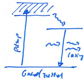
Abbildung 6.7: Die relevanten Zustände des Rubin-Lasers.
