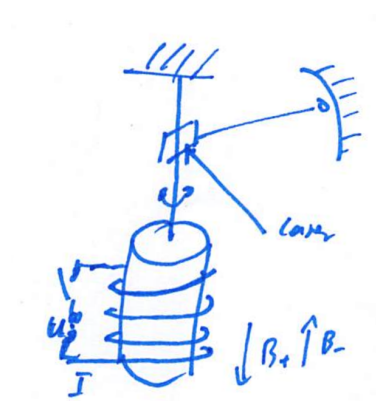
Abbildung 7.1: Einstein-de Haas-Experiment
