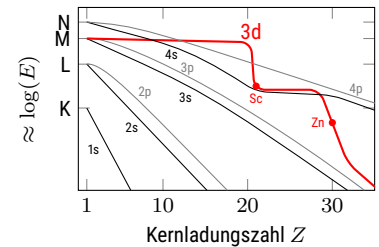
Abbildung 5.4: Schematische Verschiebung der Zustände mit steigender Kernladungszahl. Zwischen der 4s und 4p-Schale wird bei den Elementen Sc ( Z = 21 ) bis Zn ( Z = 30 ) die 3d-Schale gefüllt.
