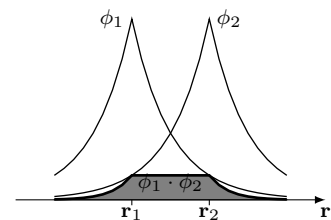
Abbildung 8.7: Skizze Überlappintegral S .
