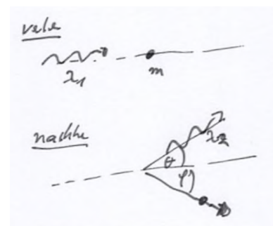
Abbildung 2.10: Kollision von Photon und Elektron.
