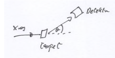
Abbildung 2.9: Versuchsaufbau zur Compton-Streuung
