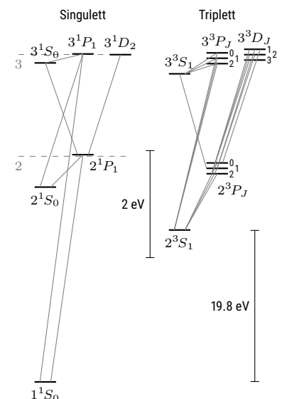
Abbildung 6.2: Termschema von Helium mit einigen erlaubten Übergängen. Man erkennt die Aufspaltung nach dem Gesamtspin. Grau strichliert die Wasserstoff-Niveaus zum Vergleich. Der 1S-Zustand ist verschoben. Die J-Aufspaltung ist vergrößert.
