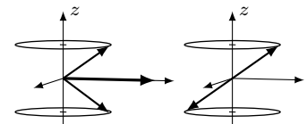
Abbildung A.4: Die Addition von zwei Vektoren |s = 1/2, m_s = 1/2\rangle und |s = 1/2, m_s = -1/2\rangle kann sowohl einen Vektor |S = 1, m_S = 0\rangle ergeben (links) als auch |S = 0, m_S = 0\rangle (rechts).
