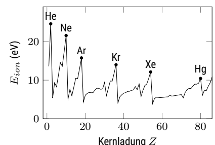
Abbildung 5.6: Ionisierungsenergie der ersten Elemente (Daten aus dem Julia-Paket Mendeleev.jl ). Die gefüllten Schalen der Edelgase sind besonders stabil.
