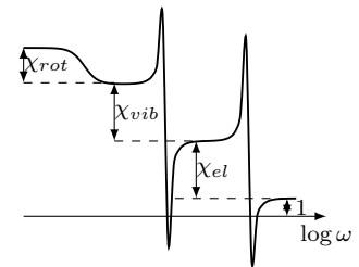
Abbildung 9.3: Addition der Suszeptibilitäten.
