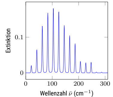
Abbildung 9.5: Das HCl-Spektrum aus Abbildung 9.4 als Extinktionsspektrum.
