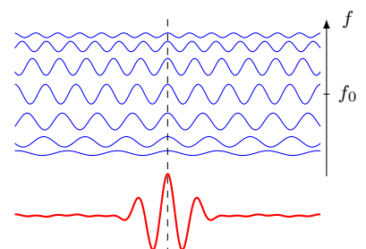
Abbildung 3.5: Synthese eines Wellenpakets
