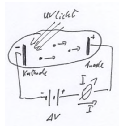
Abbildung 2.1: Skizze des Versuchsaufbaus zum Photoeffekt
