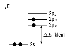
Abbildung 8.4: Elektronische Niveaus bei der Hybridisierung von Kohlenstoff.
