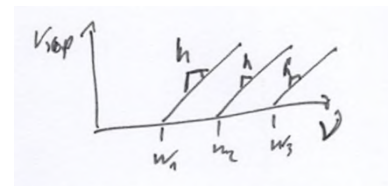
Abbildung 2.5: Stop-Spannung als Funktion der Frequenz \nu für 3 verschiedene Metalle.
