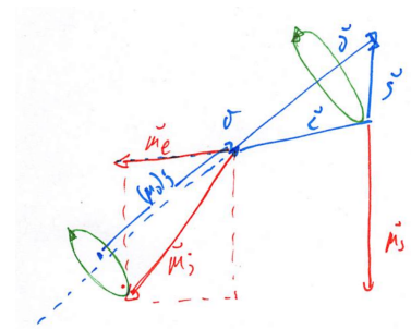
Abbildung 7.3: Der Vektor \boldsymbol{\mu}_J präzediert um \mathbf{J} , weil m_S und m_J keine guten Quantenzahlen mehr sind und g_l \neq g_s .
