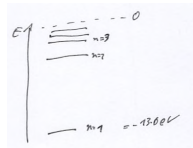
Abbildung 2.14: Zustände des Wasserstoffatoms im Bohr-Modell
