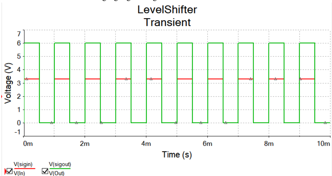
Abbildung 31: Simulation der Schaltung
