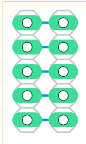
Abbildung 22: Layout Verbindungsplatine
