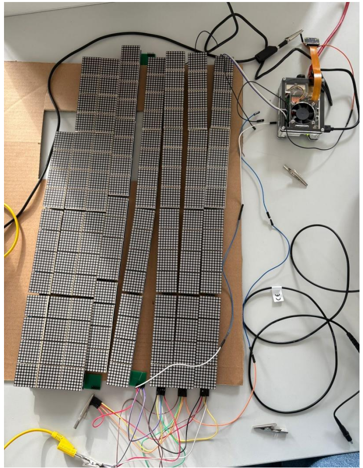
Abbildung 37: Black Mirror Setup
