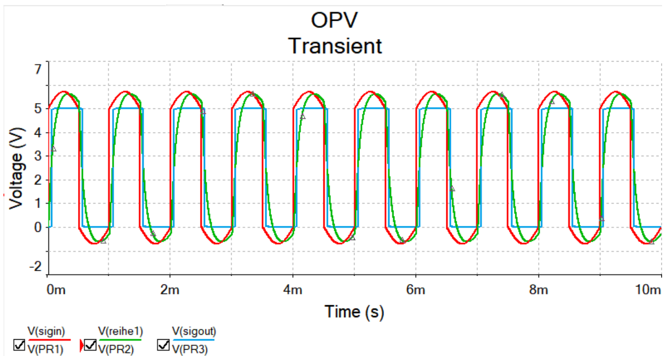
Abbildung 26: OPV-Schaltung Simulation
