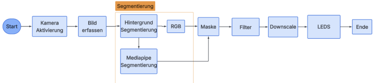
Abbildung 20: Ablaufdiagramm Personenerfassung
