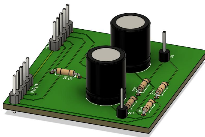
Abbildung 28: 3D Darstellung der Platine
