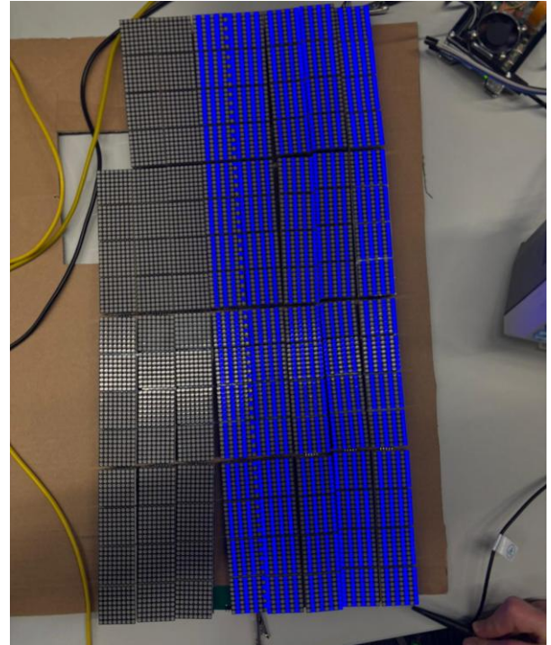
Abbildung 42: Große LED-Matrix
