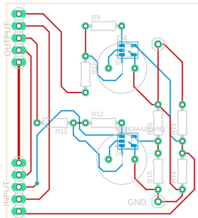
Abbildung 27: Layout der Platine
