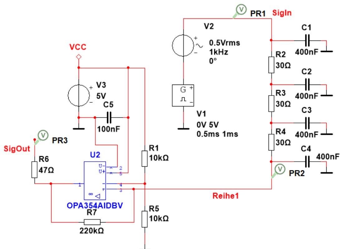
Abbildung 25: OPV-Schaltung
