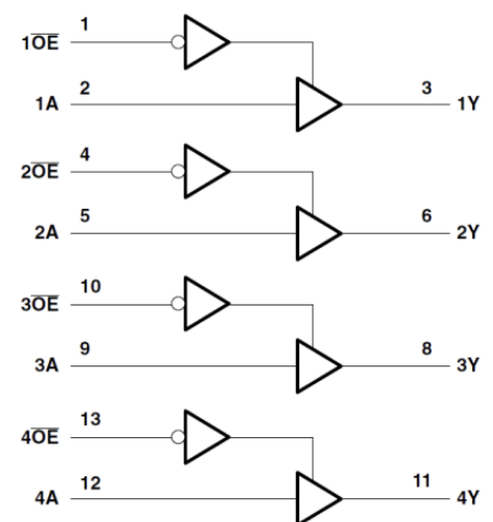
Abbildung 29: Schaltzeichen des Levelshifters [51]
