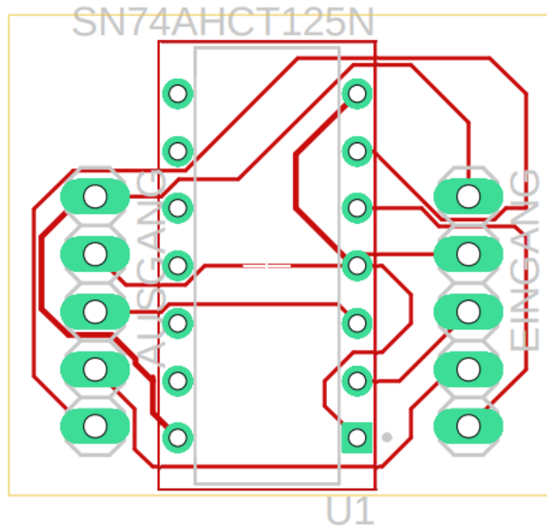
Abbildung 32: Layout der Platine
