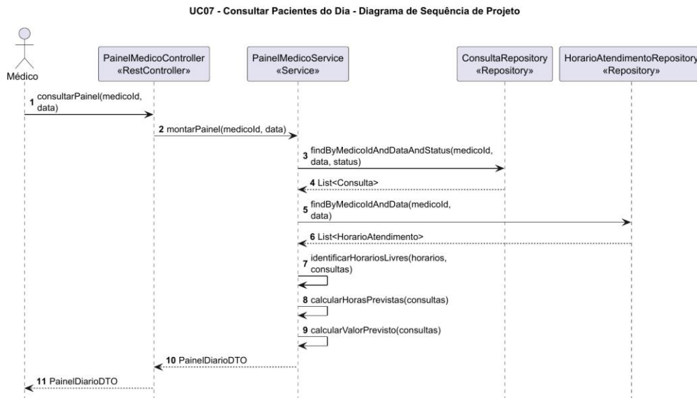
Figura 20 - Sequência de projeto do UC07 - Consultar pacientes do dia
