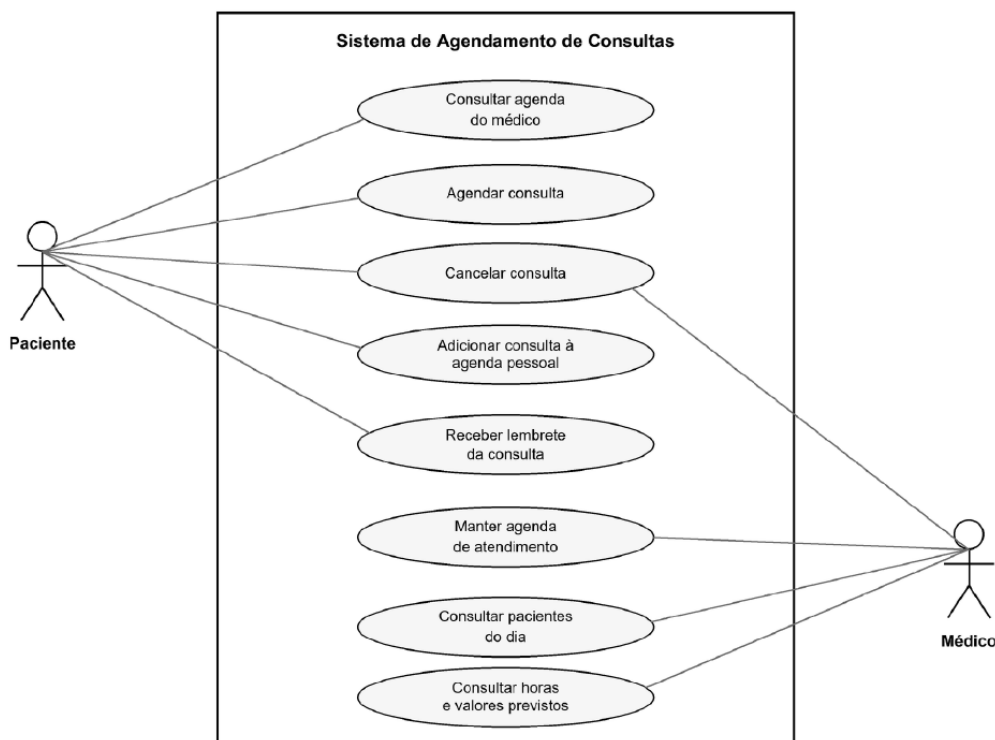
Figura 1 – Diagrama de casos de uso do Sistema de Agendamento de Consultas
