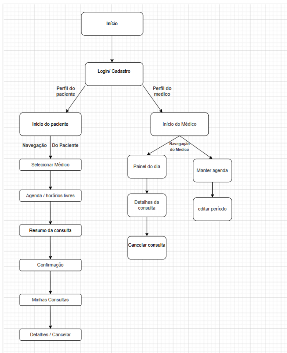
Figura 2 - Mapa de navegação do Sistema de Agendamento de Consultas
