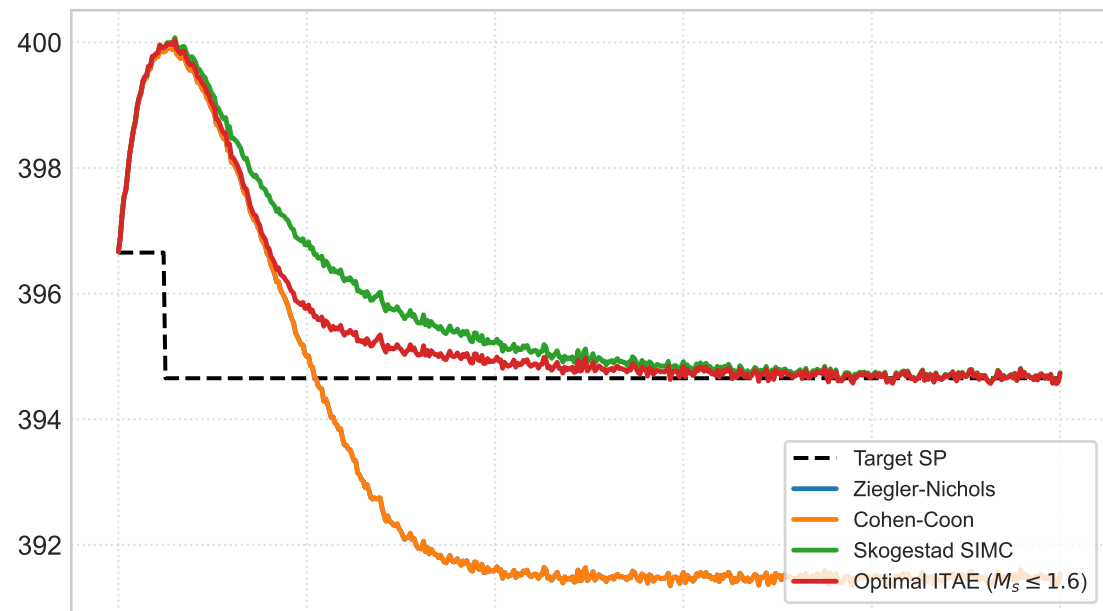
(d) Fouled Jacket (70%UA): Coolant q_j
