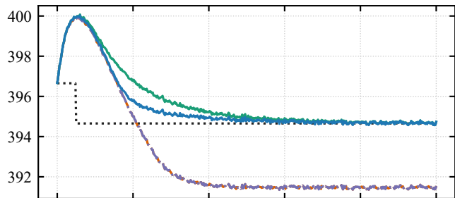
(d) Fouled Jacket (70%UA): Coolant q_j
