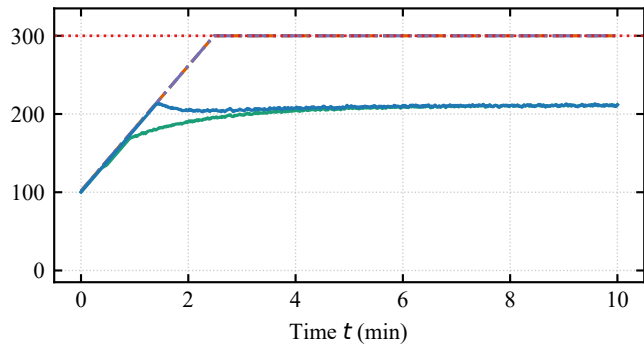
(d) Fouled Jacket (70%UA): Coolant q_j
